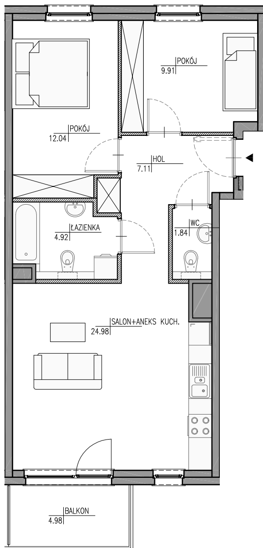
SCHEMAT LOKALU MIESZKALNEGO NA PIĘTRZE
